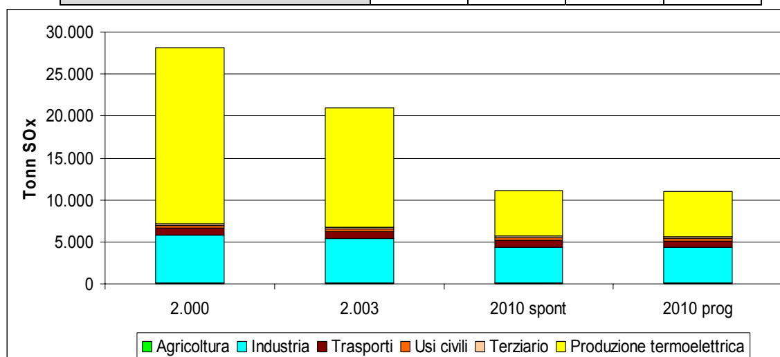
Figura 6.4 Scenari di emissione di SOx al 2010 (t)
